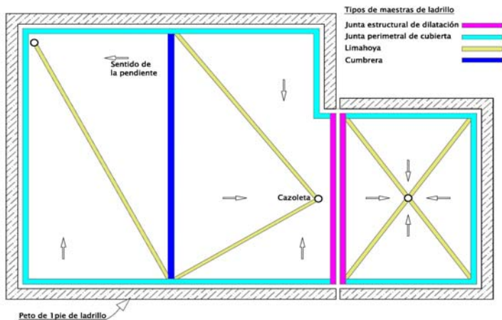
DETALLE 1a – Planta de colocación de las maestras de ladrillo (sentido de las pendientes y distribución de paños)
