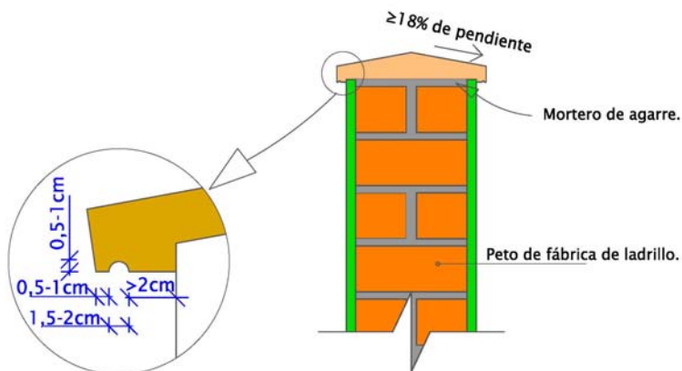
DETALLE 3a – Disposición de albardilla de piedra artificial con pendiente a dos aguas
