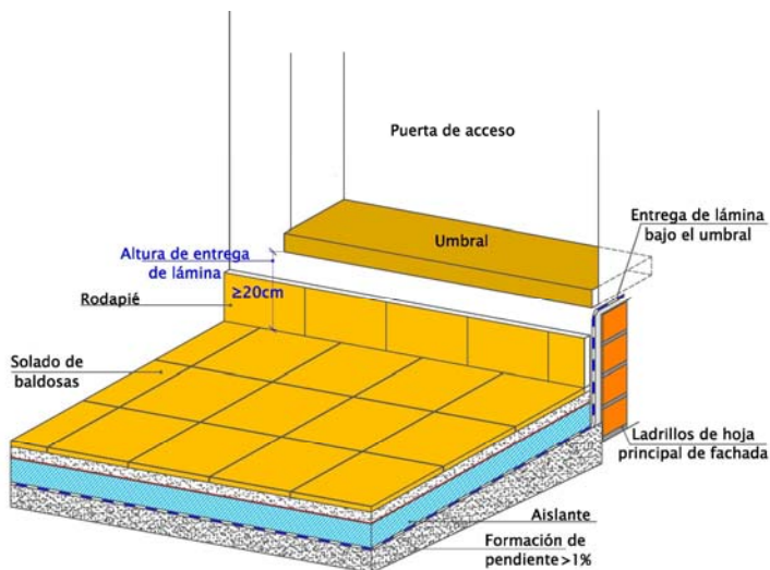
DETALLE 6a – Encuentro de la cubierta con el umbral de la puerta de acceso
