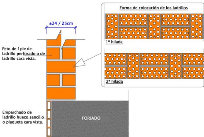
DETALLE 2a – Ejecución de peto de cubierta con fábrica de ladrillo de un pie
