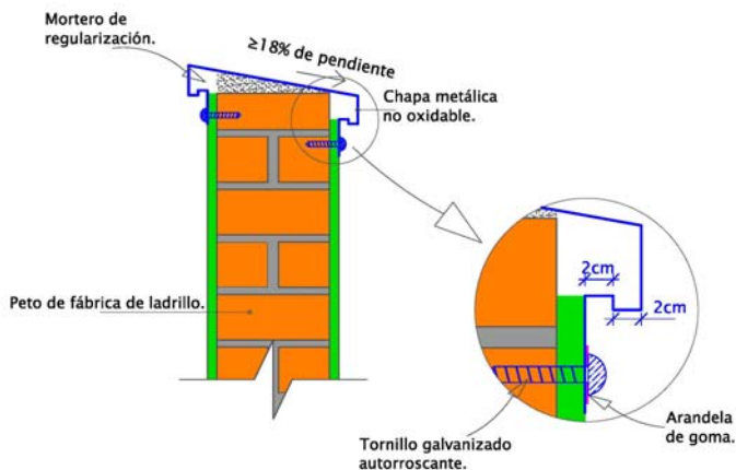
DETALLE 3b – Disposición de albardilla de chapa con pendiente a un agua
