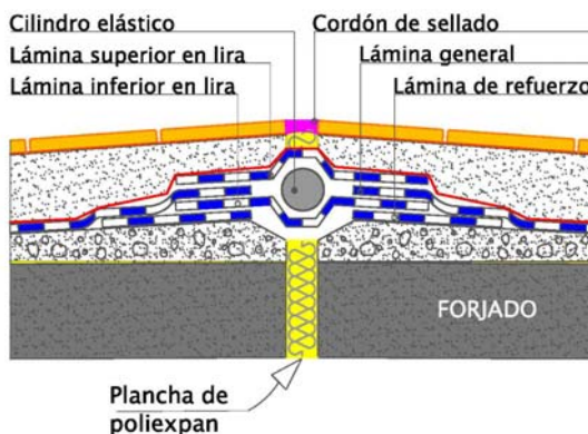
DETALLE 9b – Junta estructural de dilatación en una cubierta de tipo convencional sin aislante
