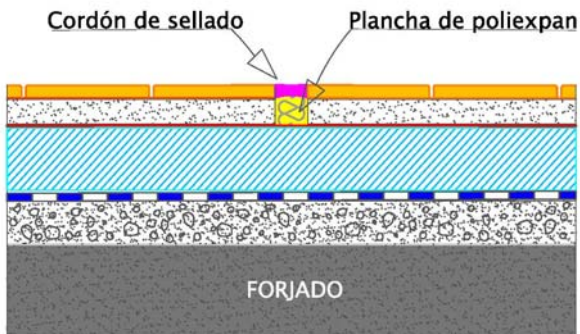
DETALLE 10b – Realización de junta de construcción-movimiento del solado
