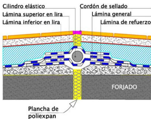
DETALLE 9a – Junta estructural de dilatación en una cubierta de tipo invertida
