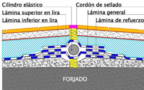
DETALLE 10a – Realización de junta de construcción-dilatación de cubierta
