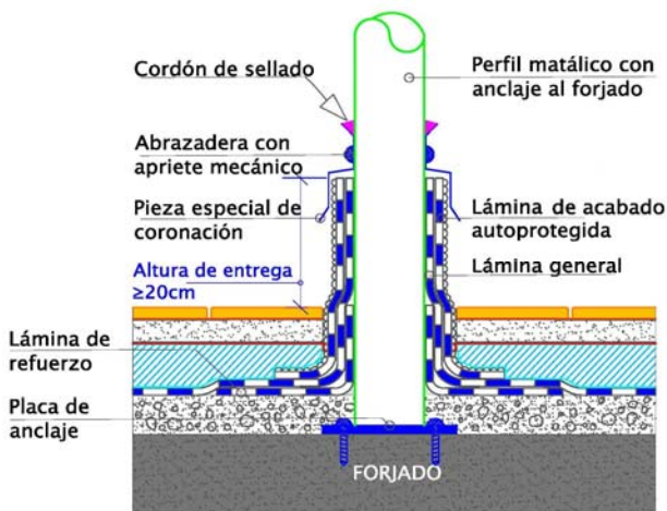
DETALLE 11b – Encuentro de la cubierta con un anclaje fijado al forjado
