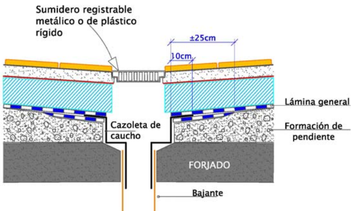
DETALLE 8b – Colocación de sumidero y cazoleta no sifónica en cubierta de tipo invertida
