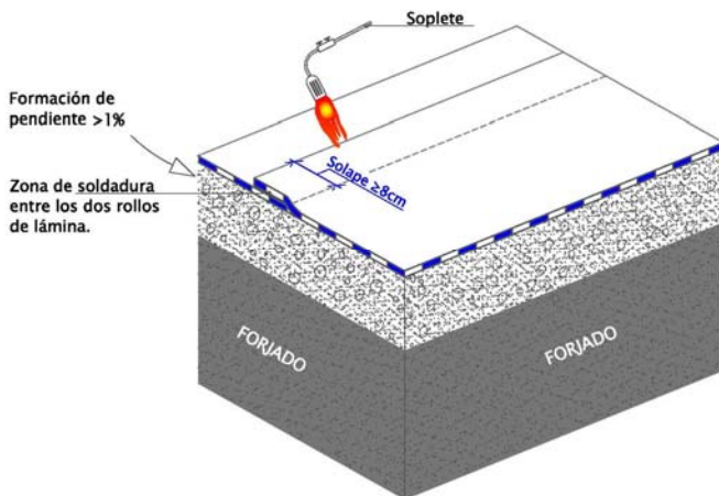
DETALLE 5a – Anchura del solape entre rollos de las láminas asfálticas
