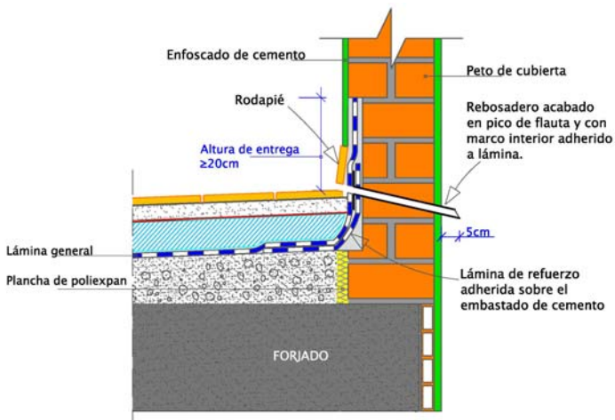
DETALLE 7b – Encuentro de la cubierta con un rebosadero
