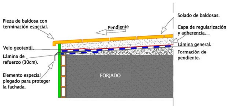
DETALLE 4b – Encuentro de la impermeabilización de un balcón con un borde libre
