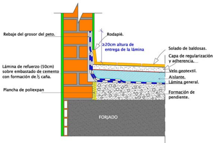
DETALLE 4a – Encuentro de un peto de fábrica de ladrillo con la cubierta
