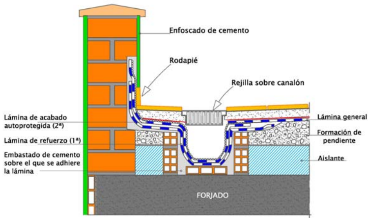
DETALLE 7a – Encuentro de una cubierta con un canalón o un sumidero lineal
