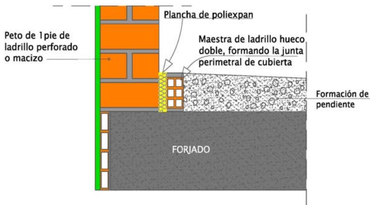
DETALLE 1b – Sección de la disposición de la maestra perimetral junto a peto
