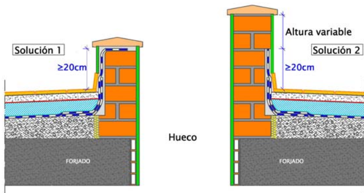
DETALLE 6b – Encuentro de la cubierta con un hueco o abertura interior
