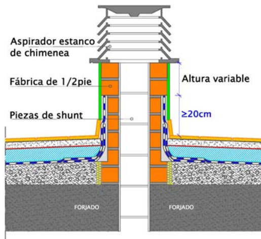
DETALLE 11a – Encuentro de la cubierta con un elemento pasante ('shunt')
