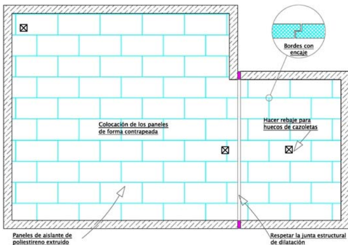
DETALLE 12a – Distribución general del aislante en los faldones de la cubierta
