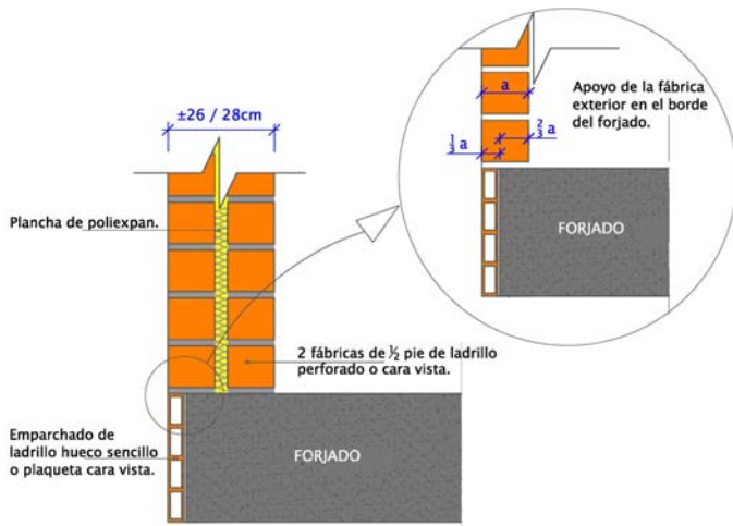
DETALLE 2b – Ejecución de peto de cubierta con fábrica de ladrillo de dos medios pies
