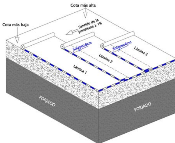
DETALLE 5b– Monte de las láminas y su disposición a cubrejuntas según el sentido de la pendiente
