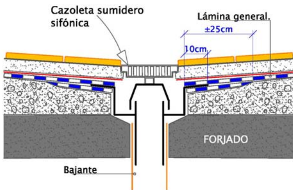
DETALLE 8a – Colocación de desagüe sifónico en cubierta convencional sin aislante
