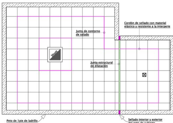
DETALLE 12b – Distribución general del solado y juntas de contorno
