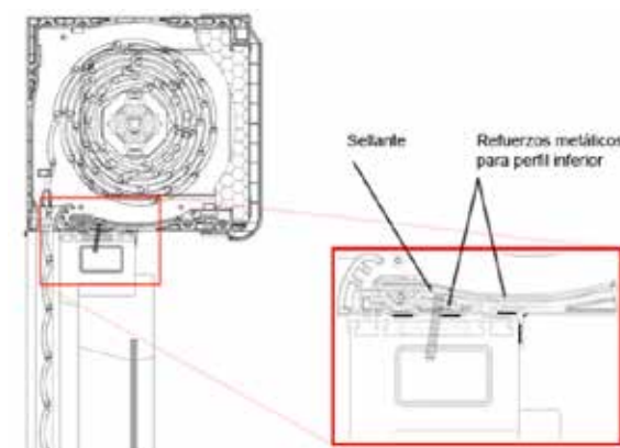
Figura 57. Detalle de unión de carpintería a cajón de persiana mediante tornillería y cajón con refuerzos metálicos para perfil inferior
